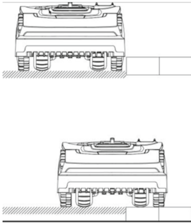
Fig. 5i
