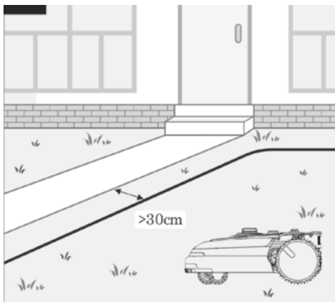
Fig. 5e
