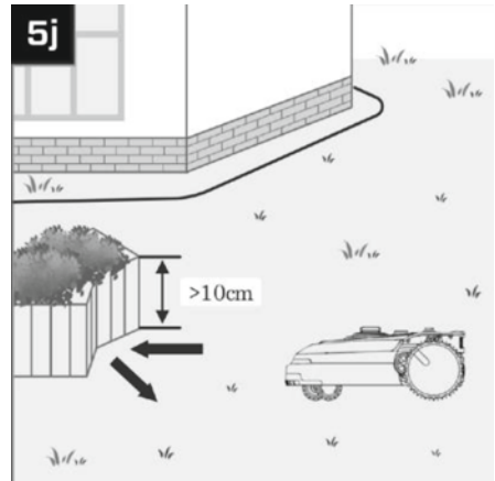
Fig. 5j
